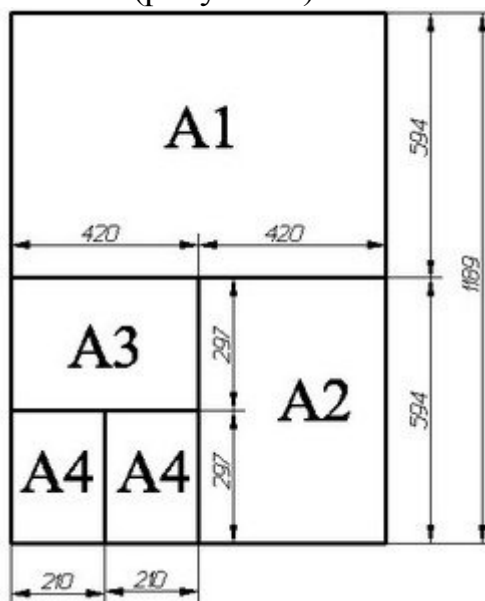
Рисунок 6 - Схема деления форматов
