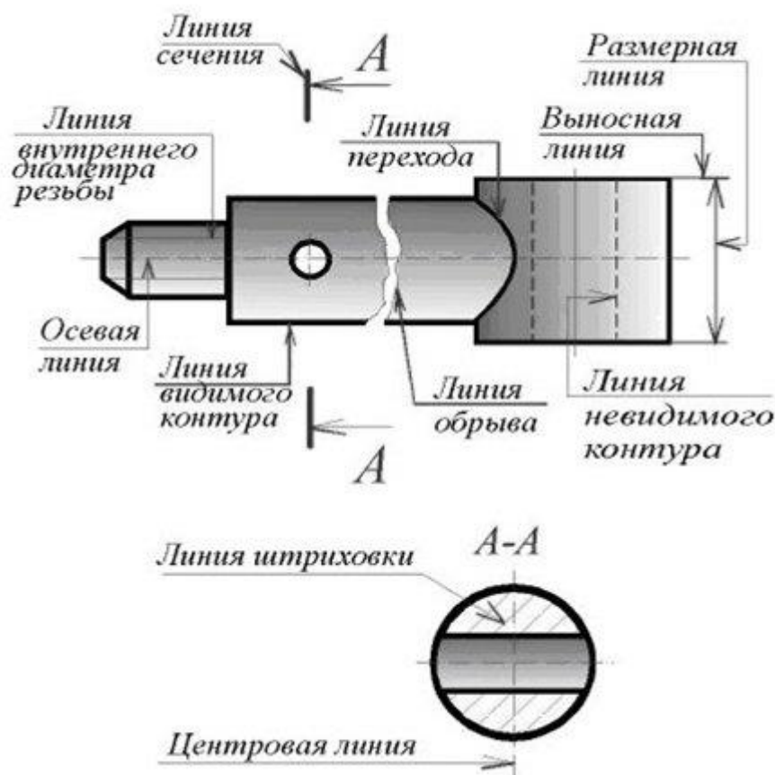
Рисунок 8 - Основные назначения линий
